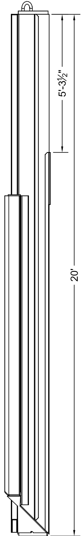
View A-A
